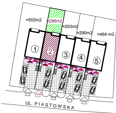
ZAGOSPODAROWANIE TERENU DZIAŁKI Skala skazona
