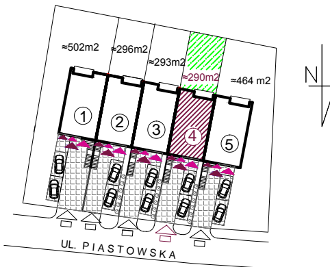
ZAGOSPODAROWANIE TERENU DZIAŁKI Skala skażona
