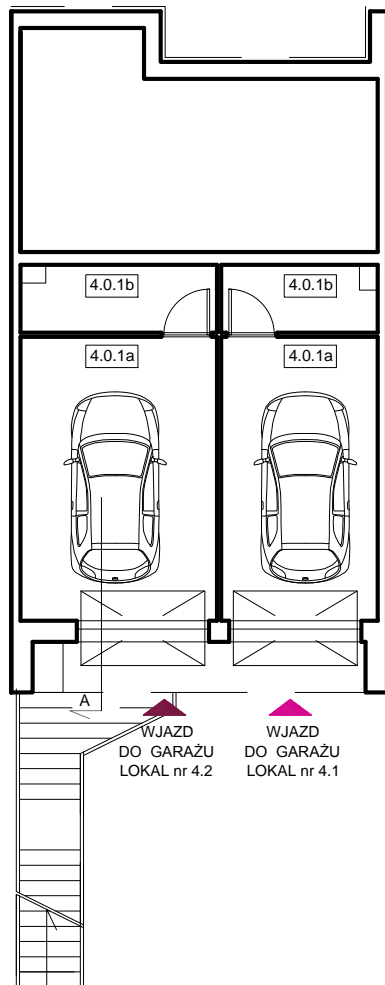
RZUT PIWNIC
