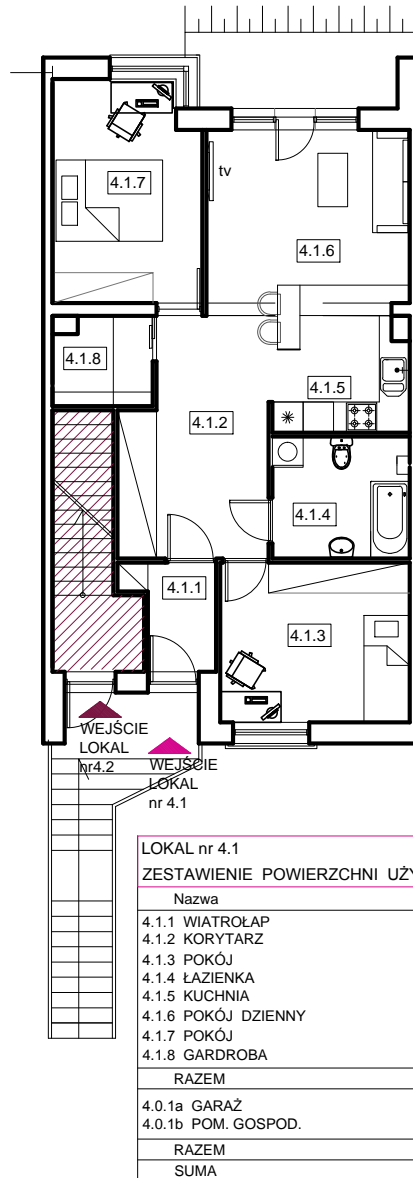
RZUT PARTERU
