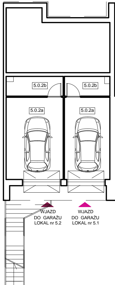
RZUT PIWNIC
